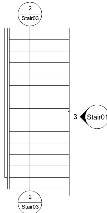
4 Stair Plan 1 : 50
