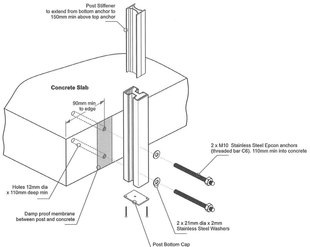
Bolt setout
