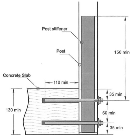
Bolt setout
